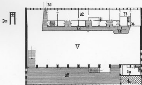
Plattegronden toekomstig station Eindhoven, na voltooiing
